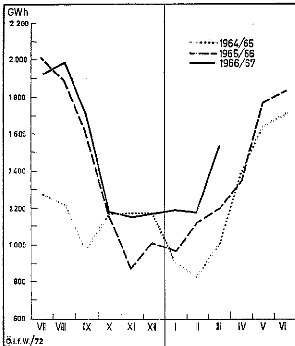
Hydraulische Stromerzeugung
