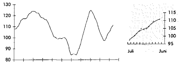
Deutschland - Industrieproduktion
