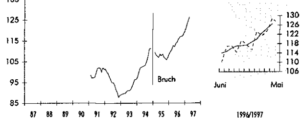
Auftragsgänge Ausland
