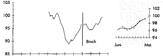
Auftragsgänge Ausland
