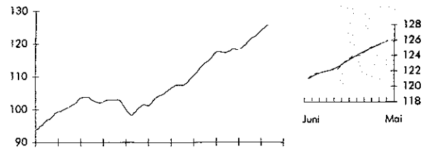
Japan - Industrieproduktion
