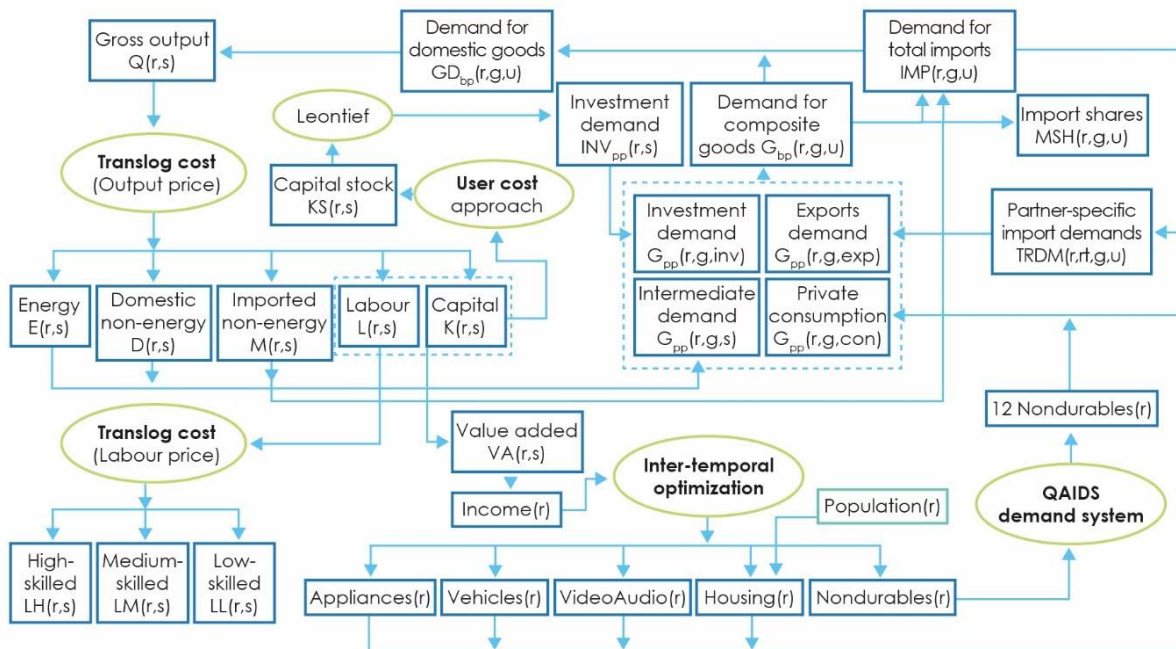
Abbildung 2: Modellstruktur ASCANIO
