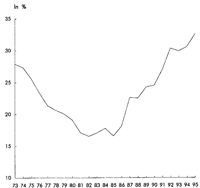
Abbildung 2: Eigenkapitalquote
