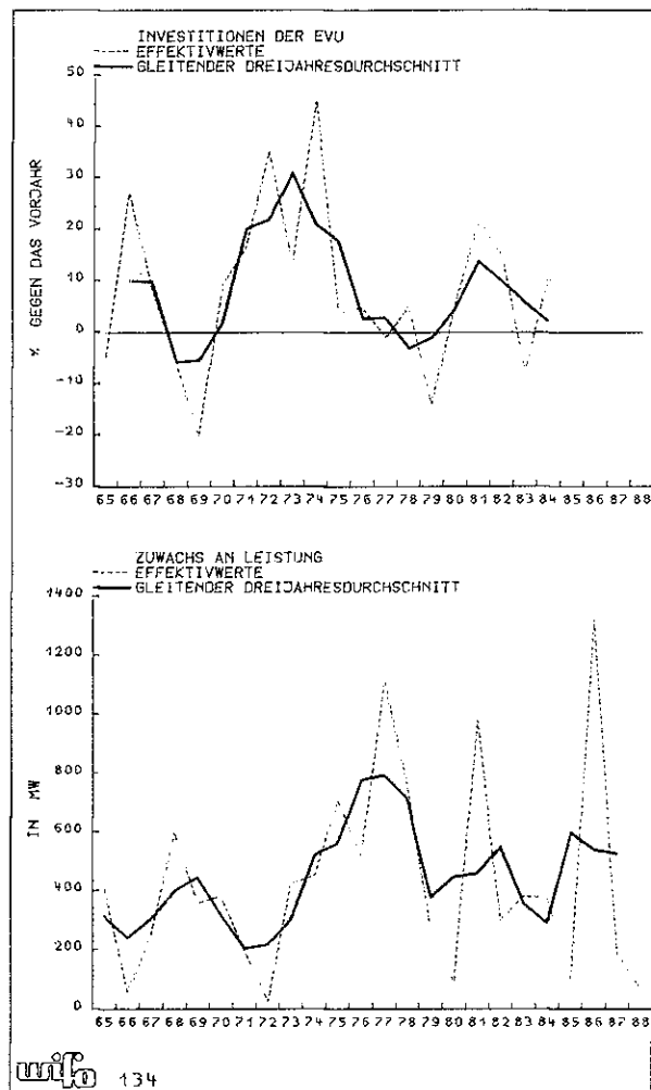
Investitionen der Elektrizitätswirtschaft und Zuwachs an Leistung
