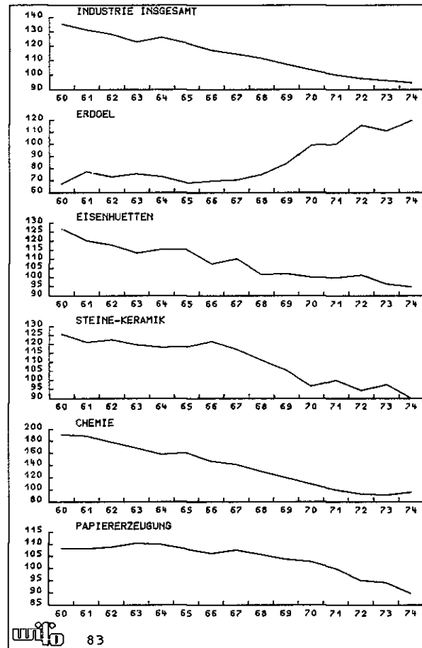
Abbildung 2 Spezifischer Energieverbrauch 1960 bis 1974 (1971 = 100)
