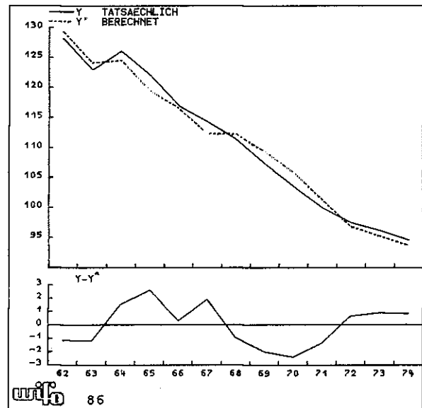
Abbildung 5 Schätzung des spezifischen Energieverbrauches (1971 = 100)
