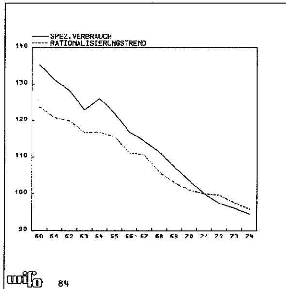
Abbildung 3 Spezifischer Verbrauch und Rationalisierungstrend 1960 bis 1974 (1971 = 100)
