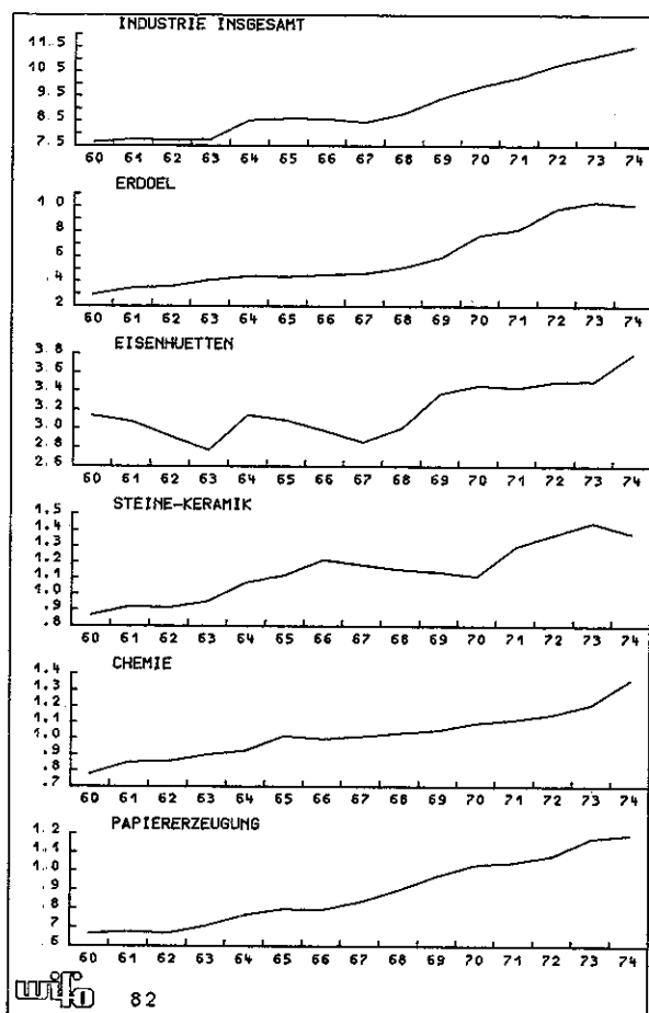
Abbildung 1 Gesamtenergieverbrauch 1960 bis 1974 (Mill t SKE)
