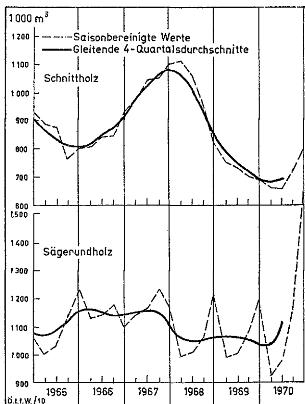
Die Lagerbewegung
