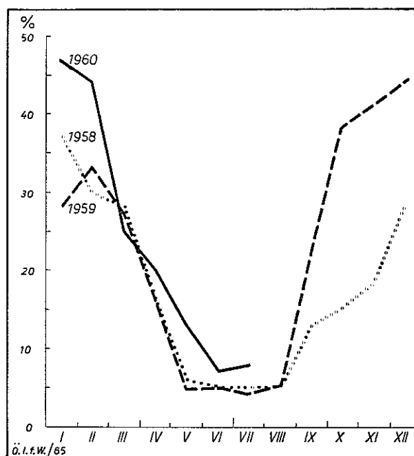
Anteil des Dampfstromes an der gesamten Stromerzeugung (Normaler Maßstab; in %)
